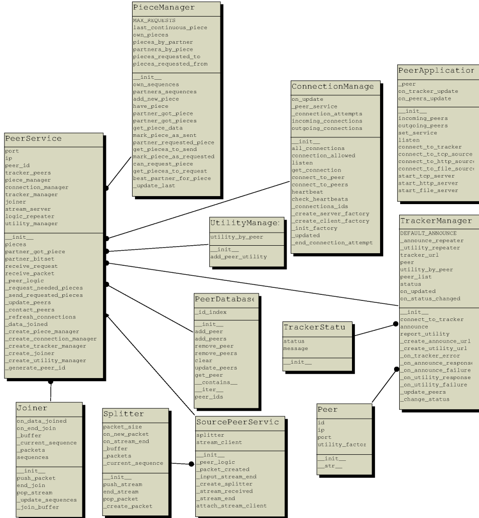
Figura A.3: Modelo de los clientes y servidores de streaming
