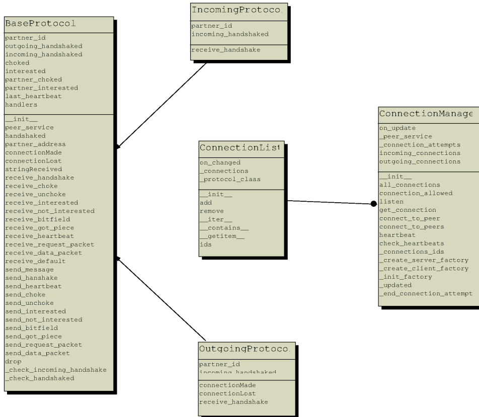
Figura A.5: Modelo del gestor de conexiones
