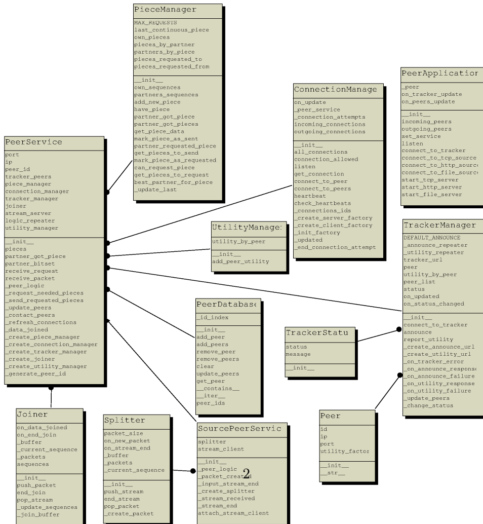
Figura A.1: Modelo de los servicios principales de Pixstream
