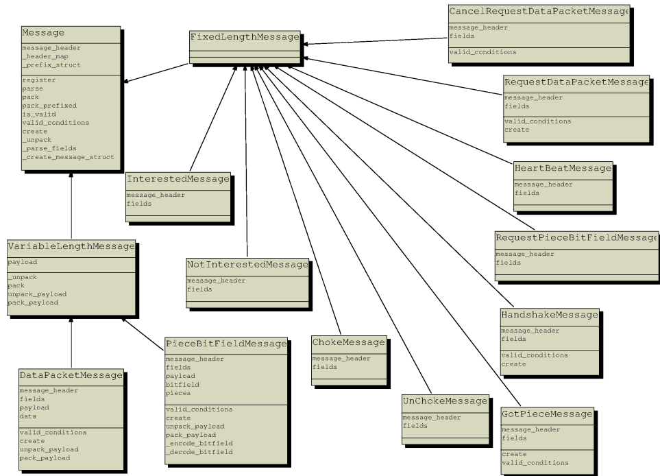
Figura A.4: Modelo de los mensajes en Pixstream
