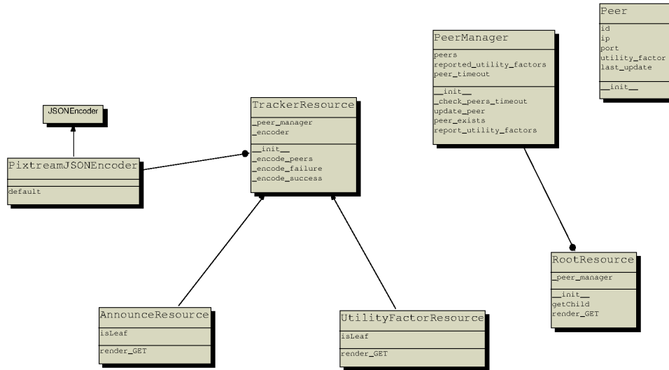
Figura A.2: Modelo del rastreador Pixtream
