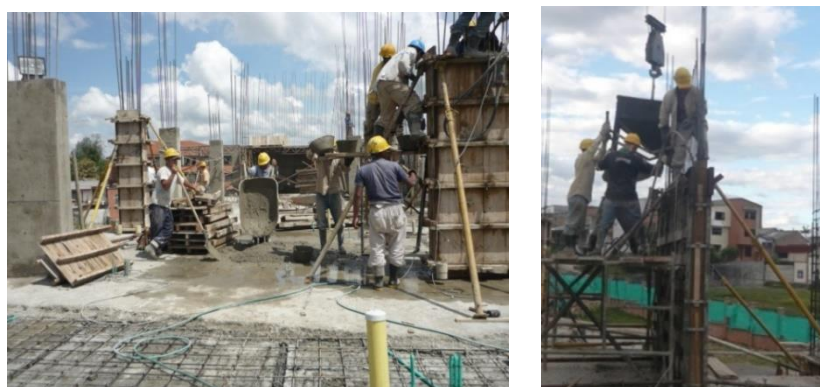
Figura N° 28. Vibrado del concreto
