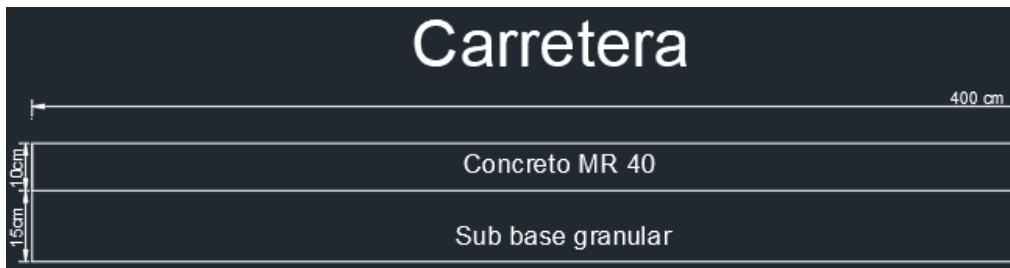
Imagen 21. Espesores de la estructura del pavimento.
