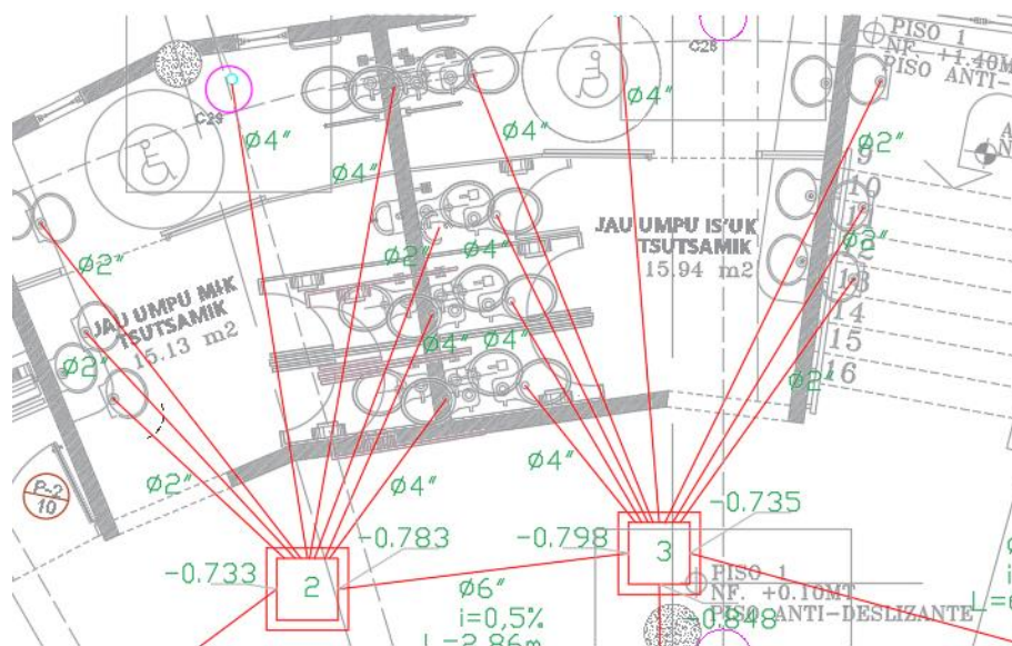
Ilustración 59. Diseño sanitario original
