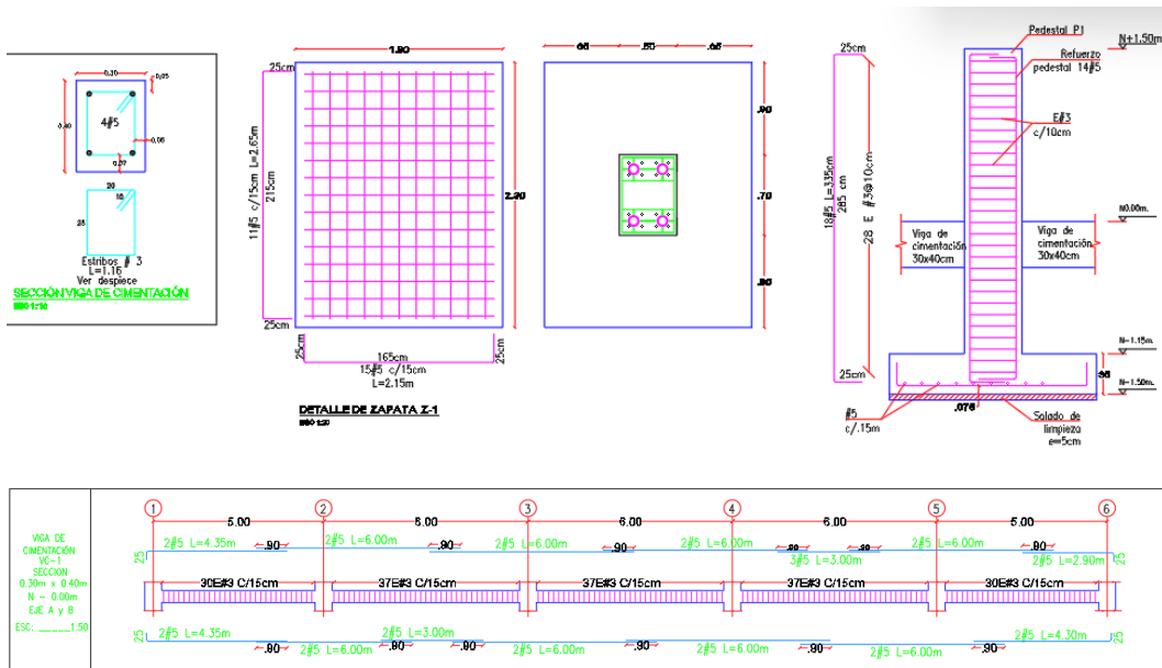
Ilustración 68. Detalles de cimentación (zapatas y viga de cimentación)
