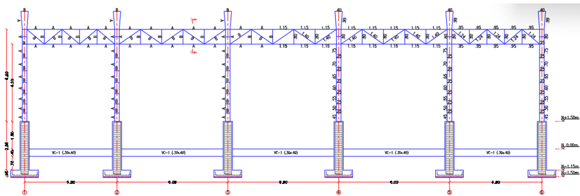
Ilustración 71. Perfil cerchas metlicas y pedestales
