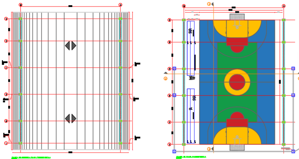
Ilustración 65. Planta de cubierta y planta de placa polideportiva
