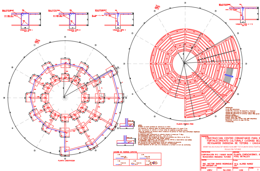
Ilustración 61. Diseño de cimentación original
