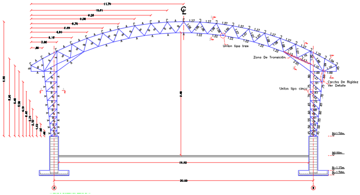
Ilustración 70. Detalle cercha metlica
