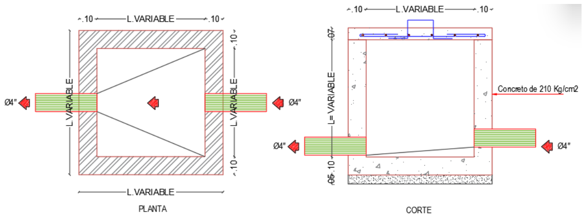
Ilustración 73. Caja de inspección.
