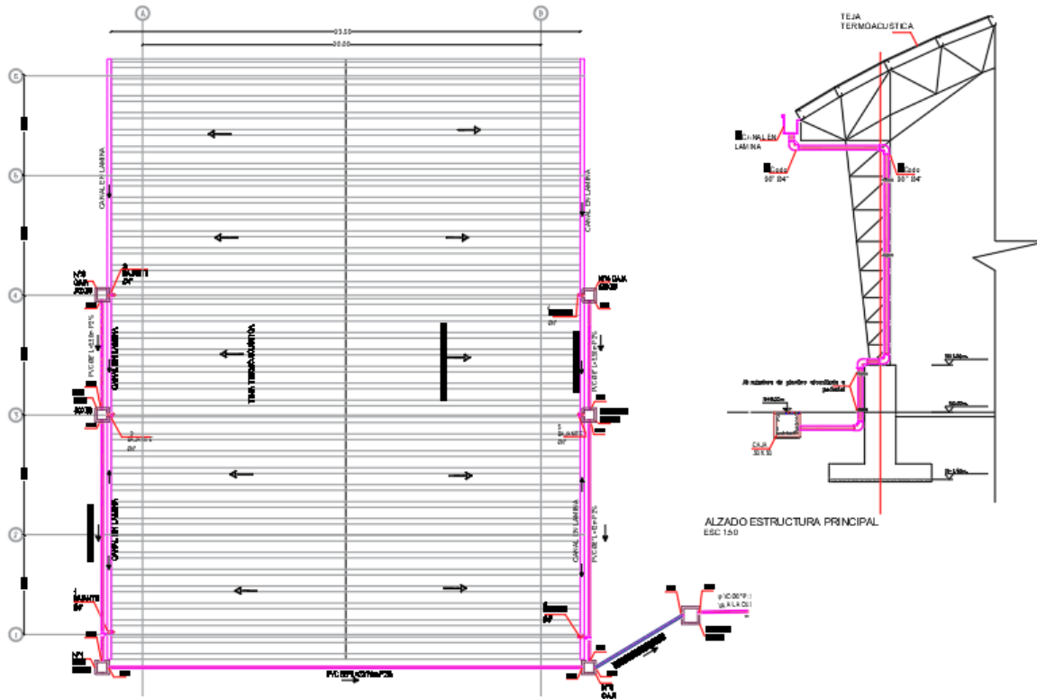
Ilustración 72. Detalles instalaciones pluviales.
