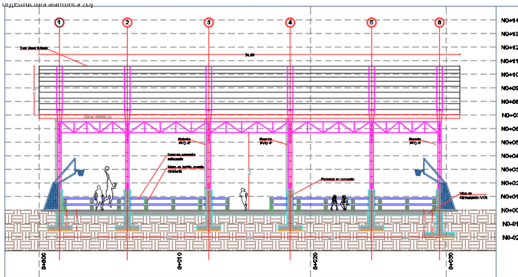
Ilustración 66. Perfil de polideportivo
