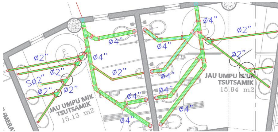
Ilustración 60. Diseño sanitario ajustado
