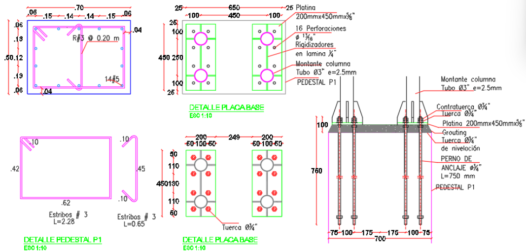
Ilustración 67. Detalles de pedestales y platinas
