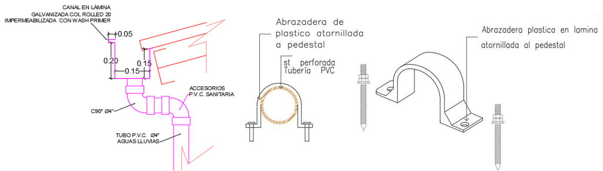
Ilustración 74. Detalle de canal y abrazaderas.
