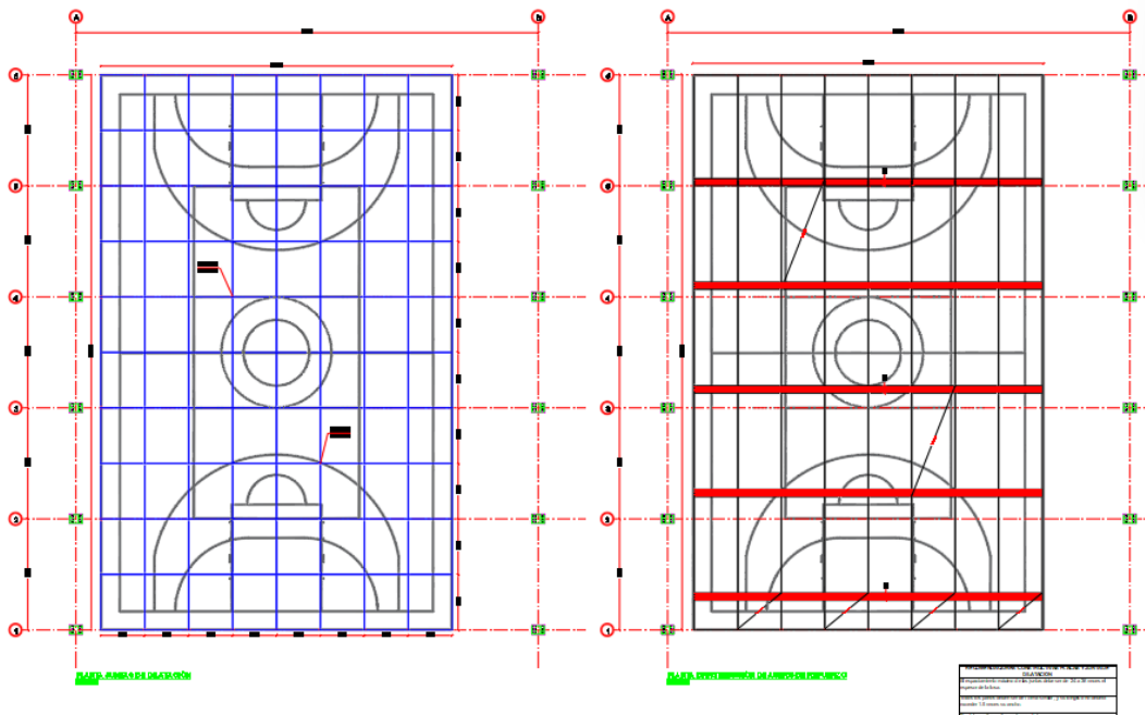
Ilustración 69. Detalle estructural placa polideportiva
