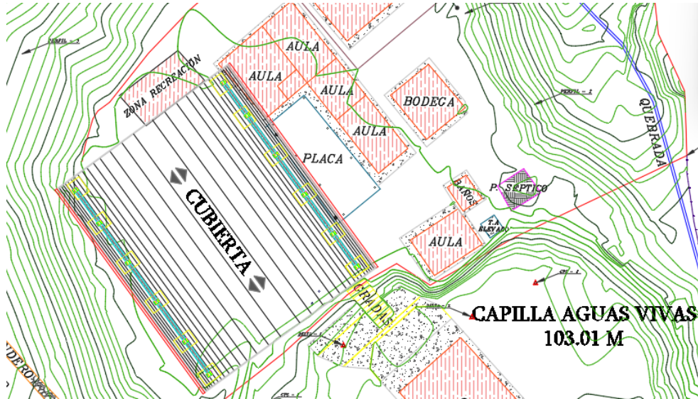
Ilustración 64. Localización de cubierta
