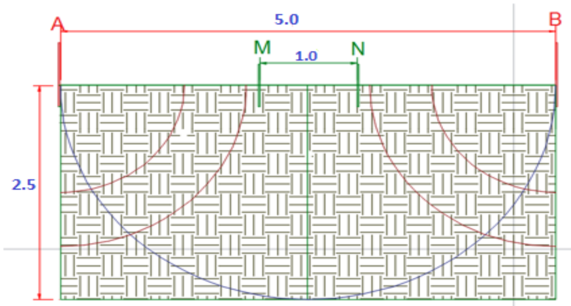
Figura 10. Esquema 2D para un sondeo a 2.5 metros de profundidad
