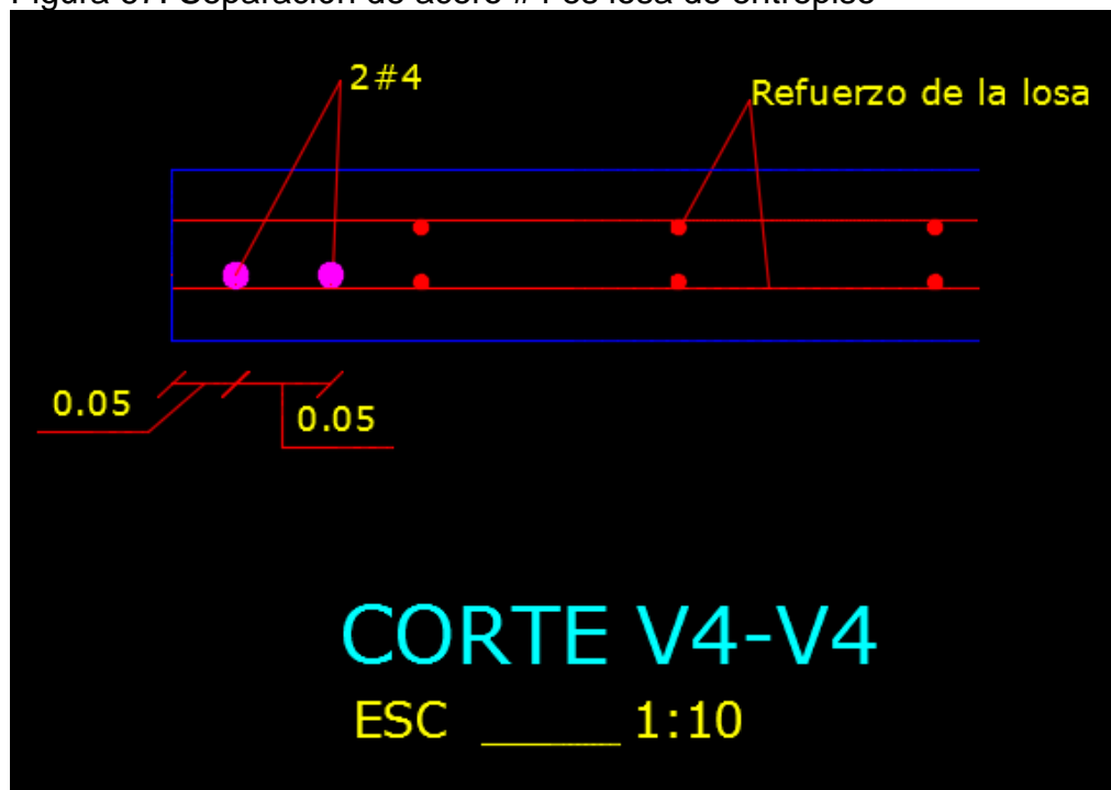
Figura 67. Separación de acero #4 es losa de entrepiso
