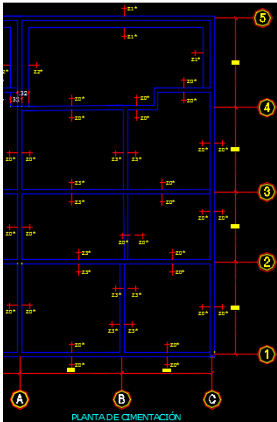
Figura 28. Plano 13/25 acero de cimentación
