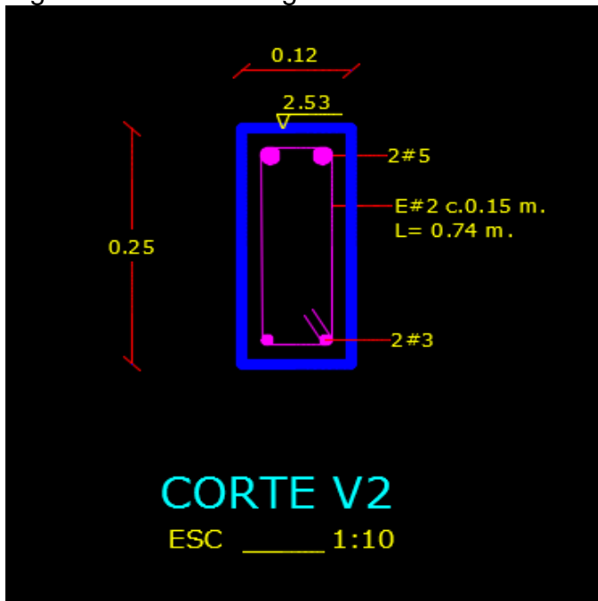
Figura 66. Corte de viga en voladizo V2
