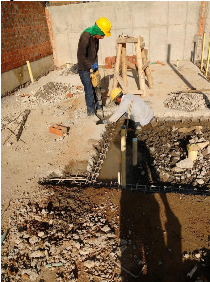
Figura 49. Demolición losa de cimentación casas 13A y 14A
