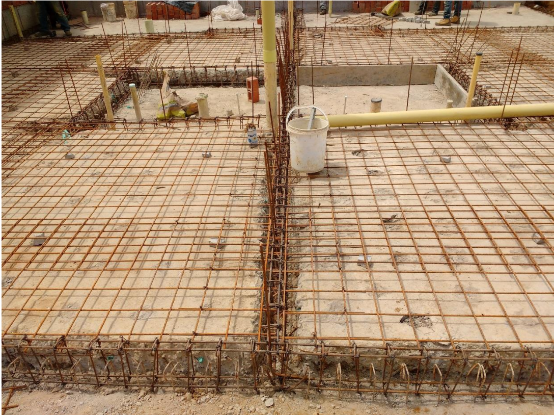
Figura 50. Armado de acero en parte superior losa de cimentación casas 13A y 14A
