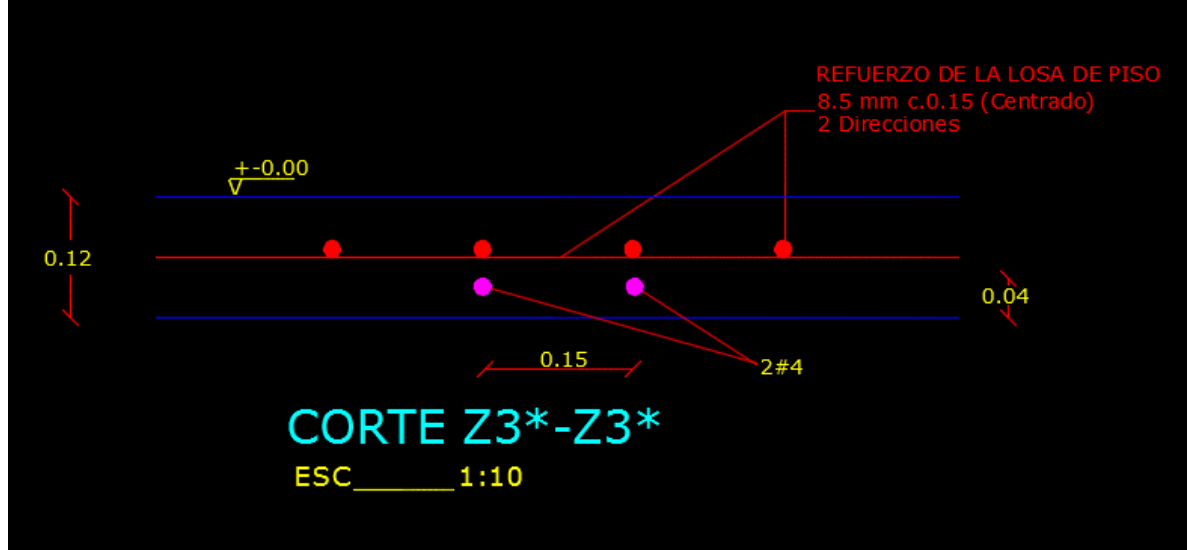
Figura 29. Ubicación de acero de refuerzo a flexión
