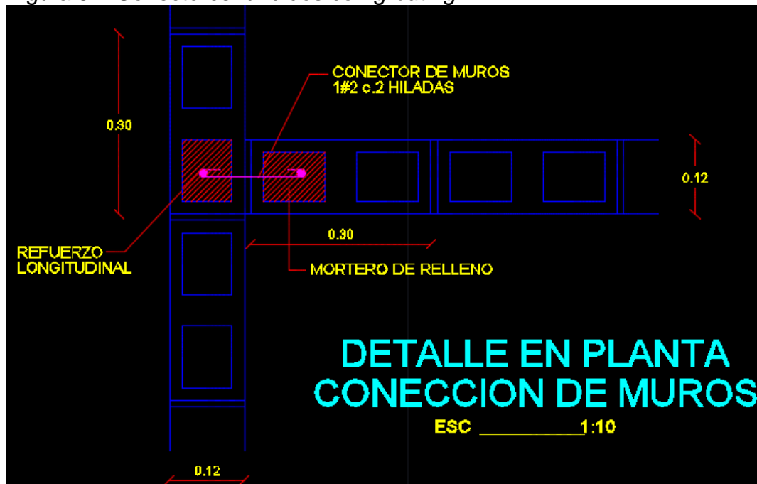
Figura 57. Conectores fundidos con grouting .
