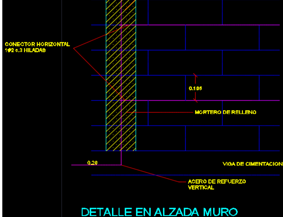
Figura 58. Ubicación de grafiles (refuerzo horizontal)
