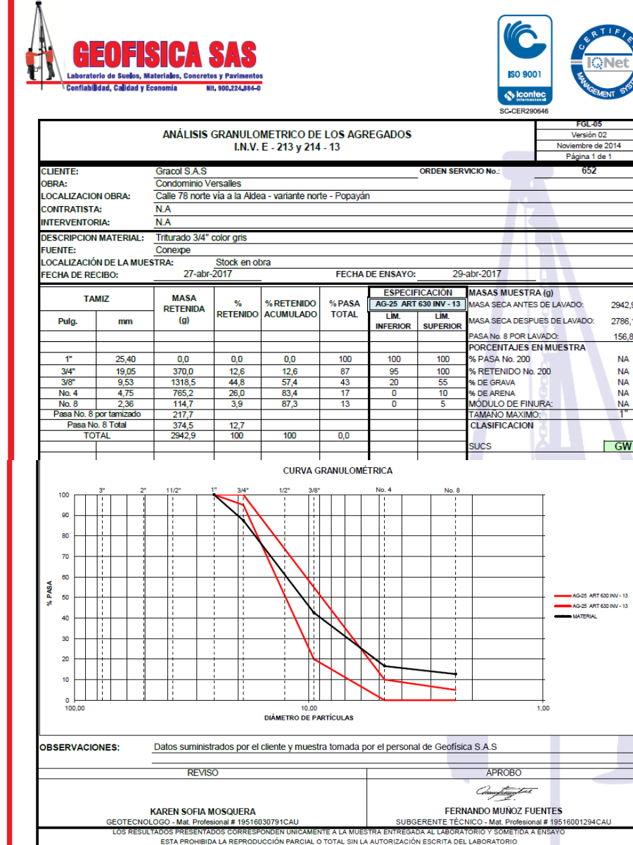
Figura 14. Granulometría agregado grueso 3/4"
