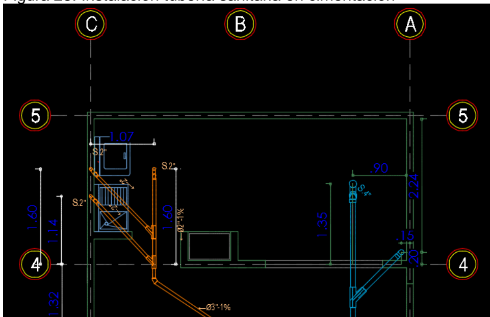
Figura 25. Instalación tubería sanitaria en cimentación
