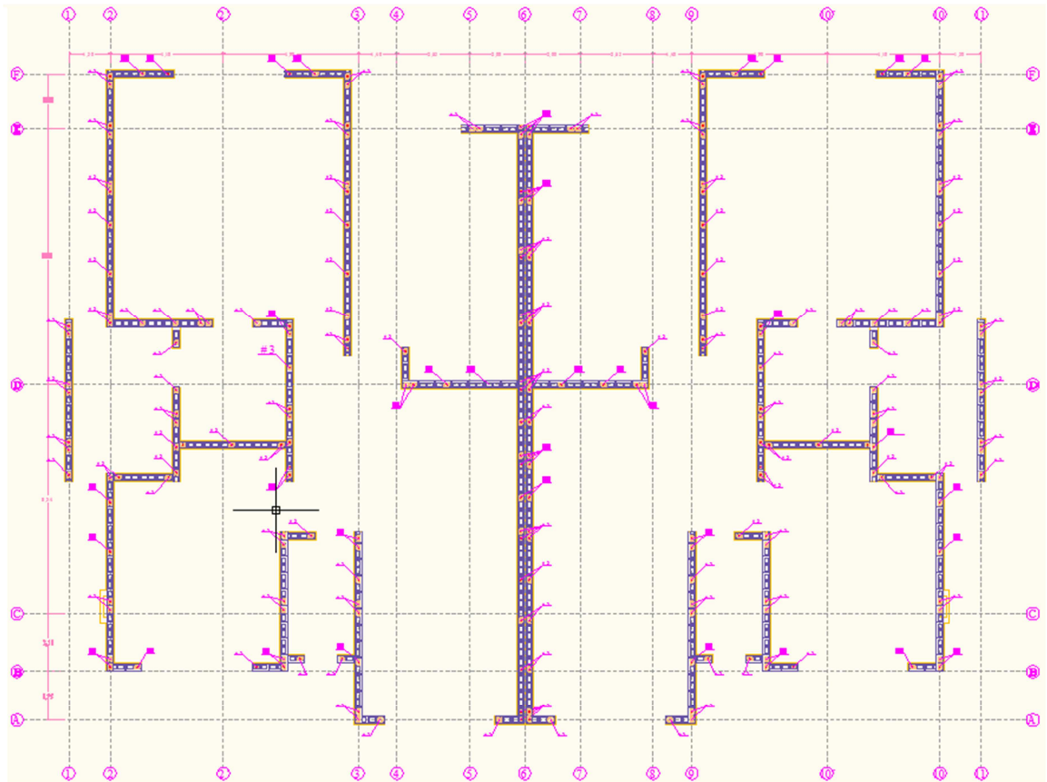
Figura 25. Planta muros segundo piso.
