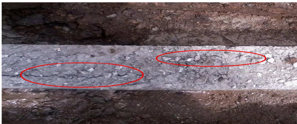
Figura 45. Falla por retracción y temperatura del concreto.
