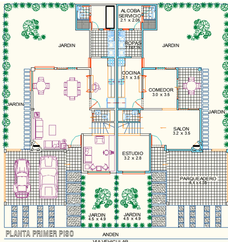
Figura 2. Plano arquitectónico primer piso.
