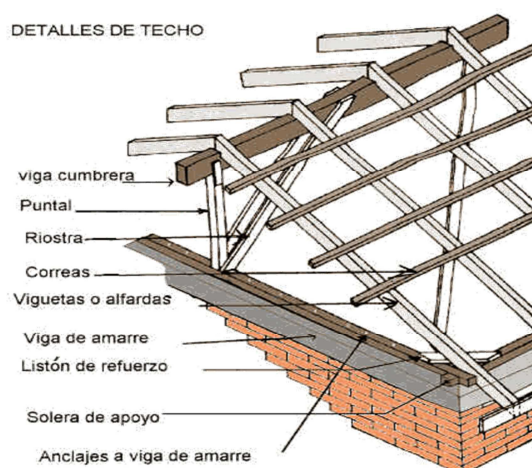
Figura 37. Elementos de cubierta.
