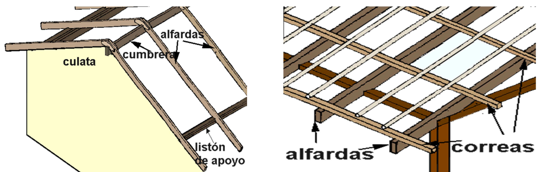
Figura 40. Ilustración de Alfardas y correas.
