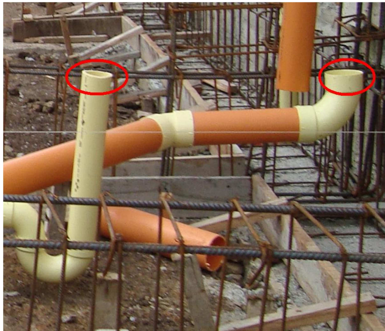
Figura 48. Tubería de desagüe sanitario sin protección.
