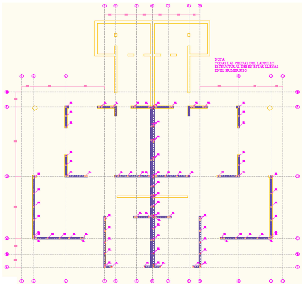
Figura 24. Planta muros primer piso.
