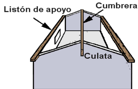
Figura 39. Ubicación de listón de apoyo y cumbrera.
