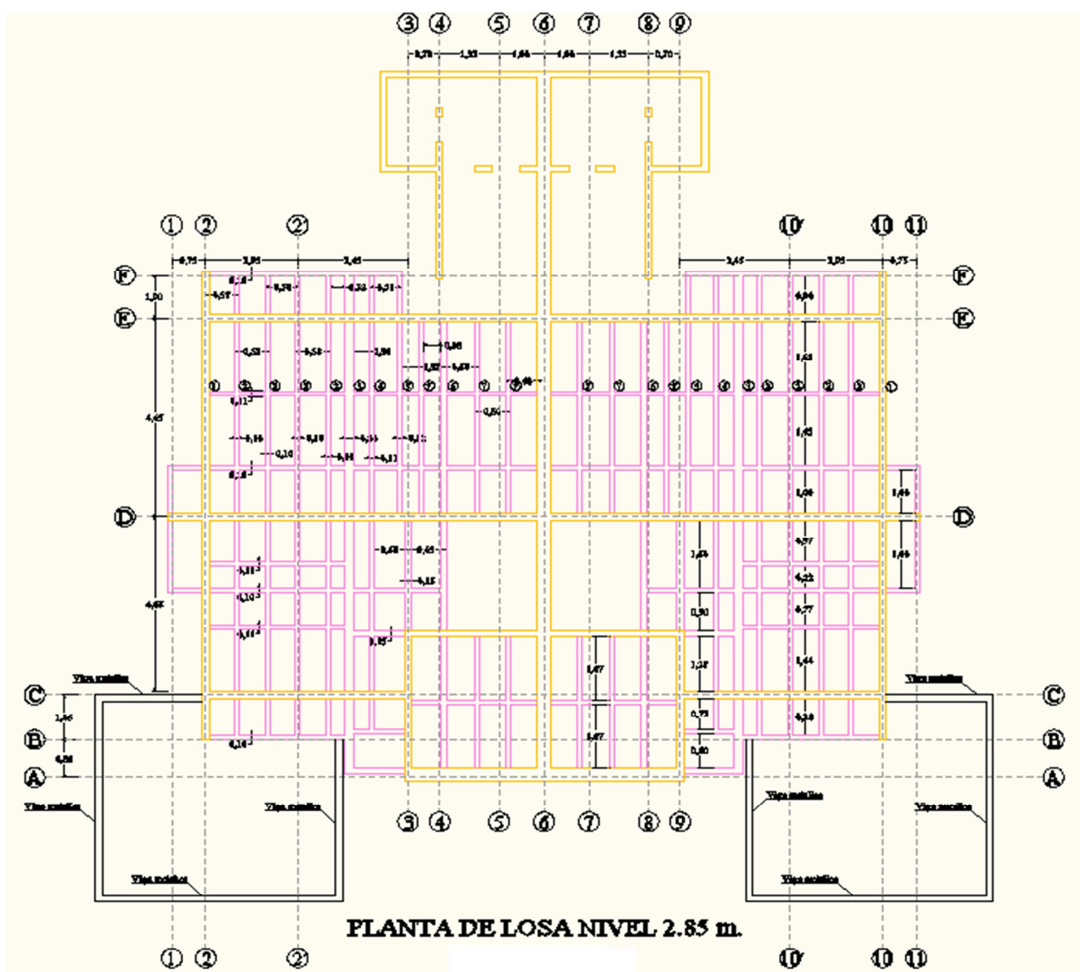
Figura 33. Plano en planta de losa.
