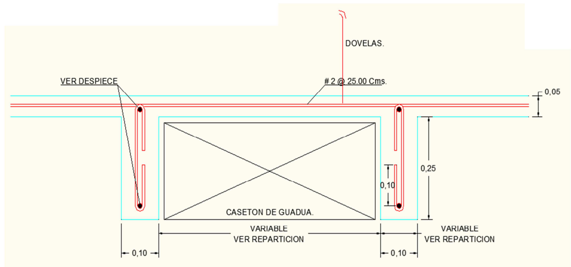
Figura 26. Corte transversal de la losa de entrapiso.
