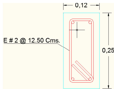
Figura 34. Sección transversal viga de cubierta.
