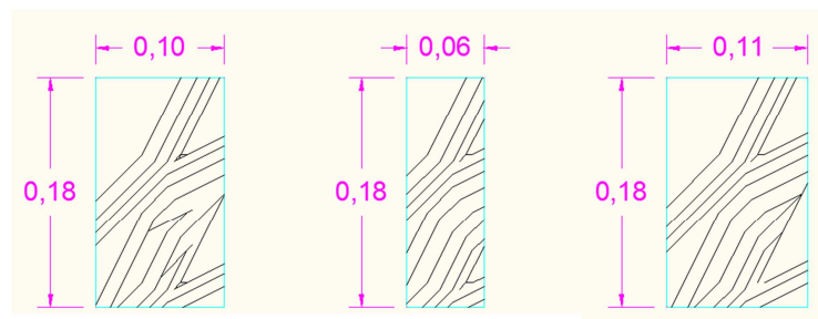
Figura 38. Sección transversal de vigas de madera de cubierta.
